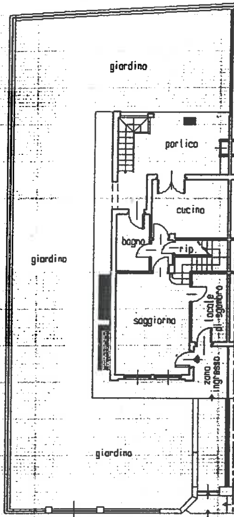
PIANTA PIANO TERRENO h. m. 2.80
