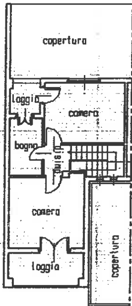
PIANTA PIANO PRIMO h. m. 2.80
